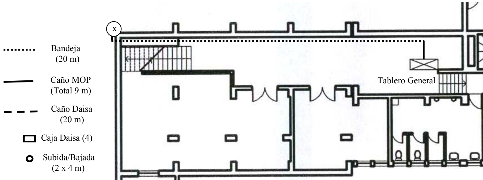
SUBSUELO
