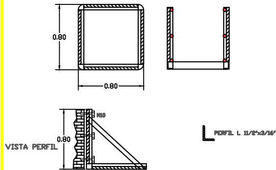
Estructura de Perfil L para base de apoyo para las Unidades Exteriores de Aires
