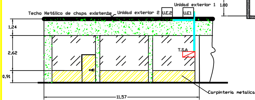
Estructura de Perfil L para base de apoyo para las Unidades Exteriores de Aires
